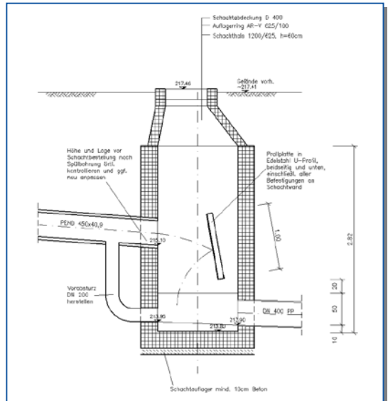
Schnitt Schacht mit Pallplatte
